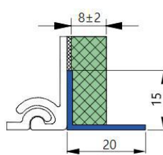
Ometni kotnik za ekstrudirane sisteme
