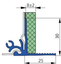
Ometni kotnik za valjane sisteme *Opcijsko se lahko kotnik prireže
